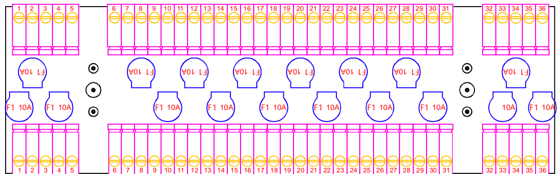
BORNERO DE CONEXIONES REF: 141005F
