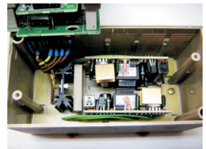
Posición dentro de la caja del autómata
