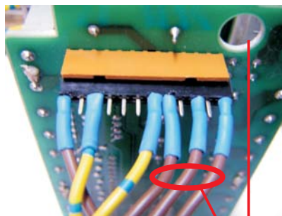
Posición del conector. Los tres cables marrones a la parte del derecha
